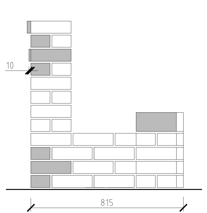
END ELEVATION
