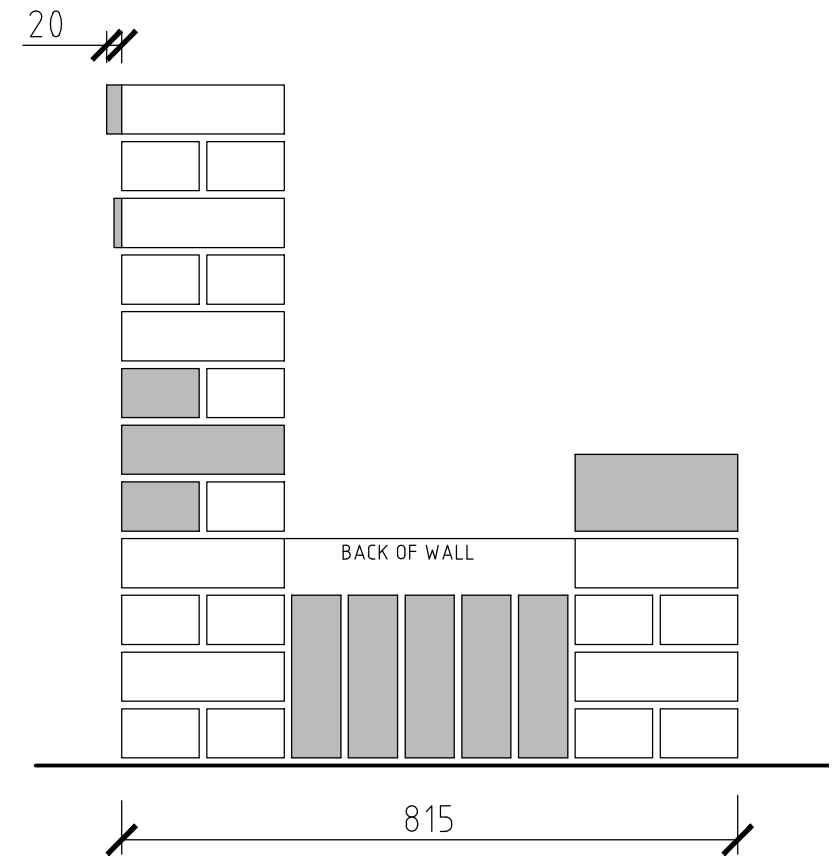
END ELEVATION
